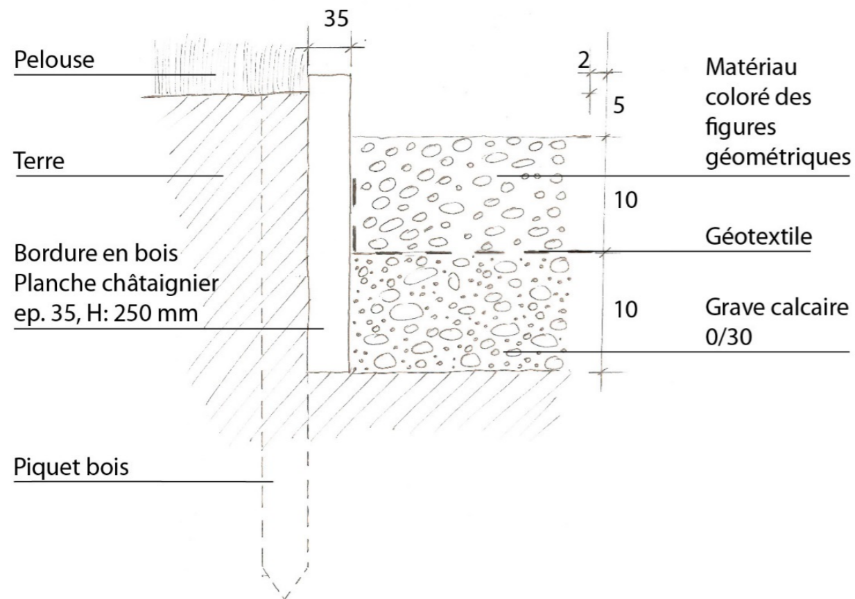
Coupe de principe 1 : mise en place de la bordure en bois
