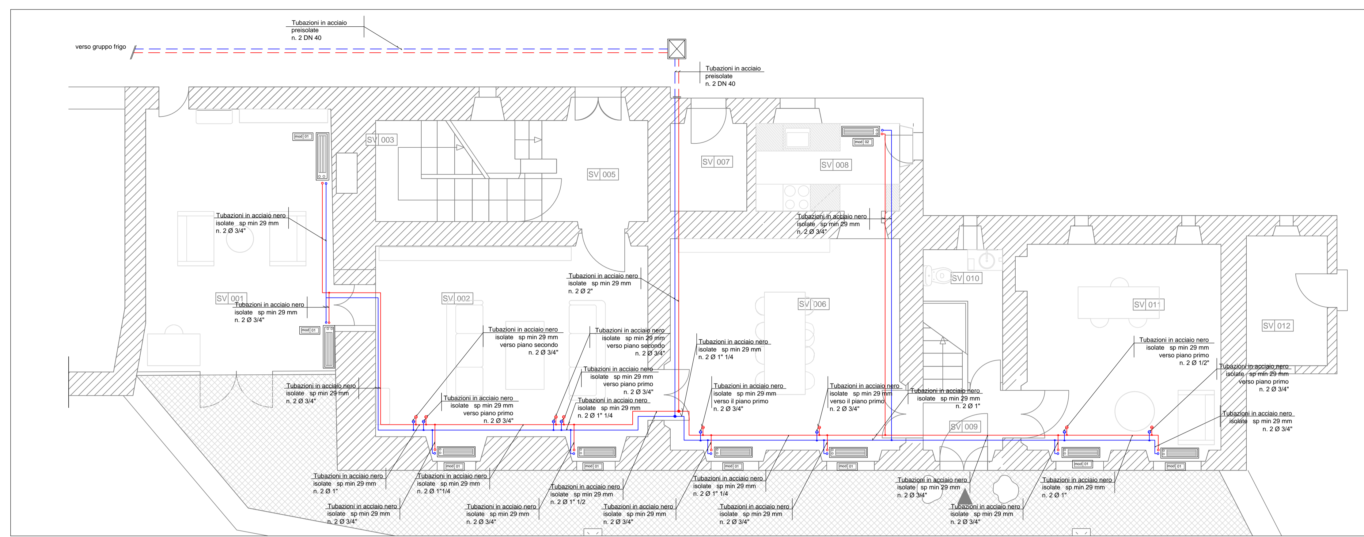
Pianta Piano Terra - linea freddo per raffreddamento
