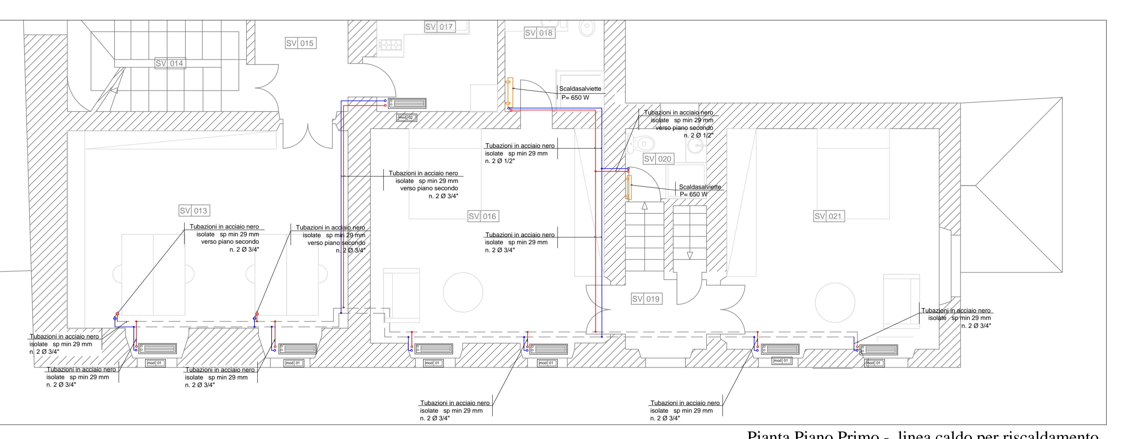
Pianta Piano Primo - linea caldo per riscaldamento
