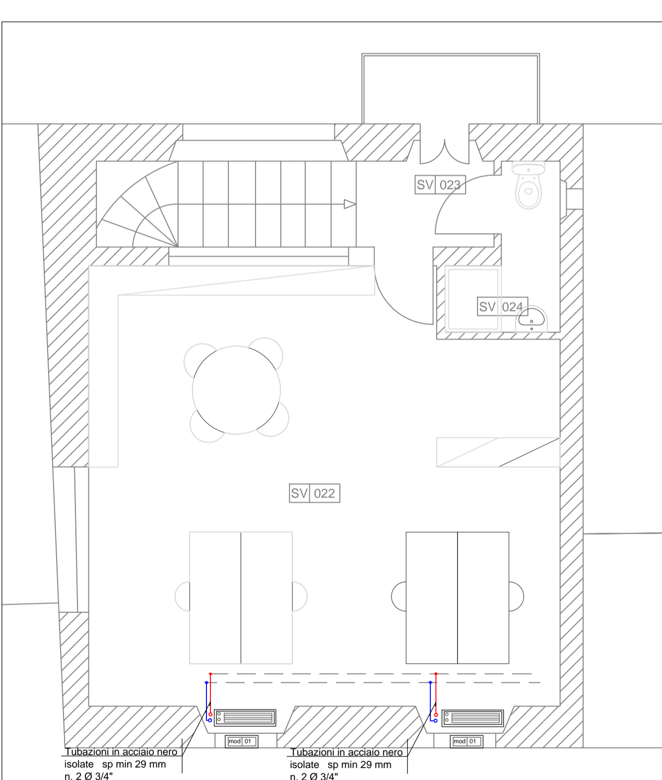
Pianta Piano Secondo Linea freddo per raffreddamento
