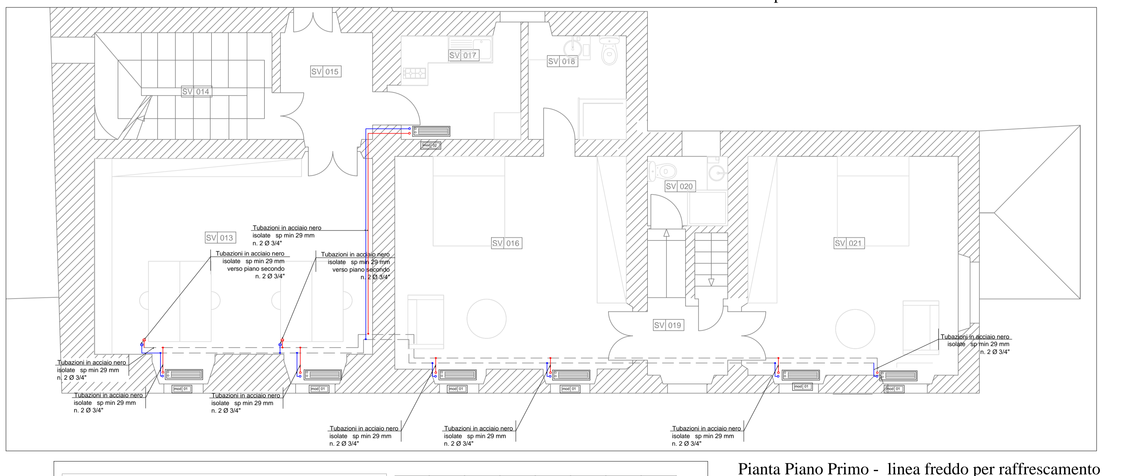
Pianta Piano Primo - linea freddo per raffreddamento
