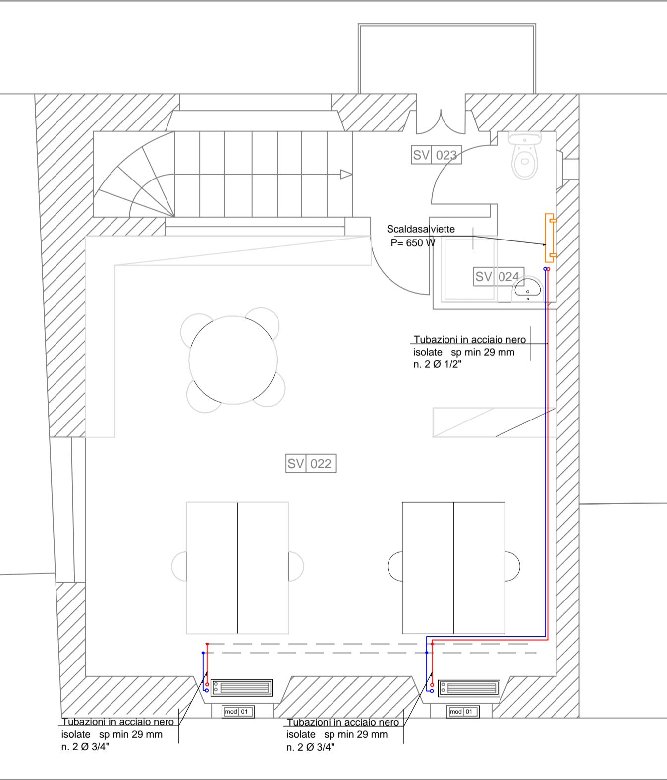
Pianta Piano Secondo Linea caldo per riscaldamento
